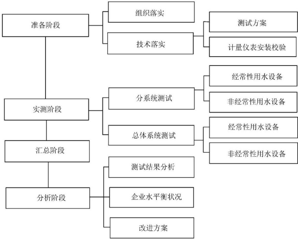
图 1-1 水平衡测试工作程序图
